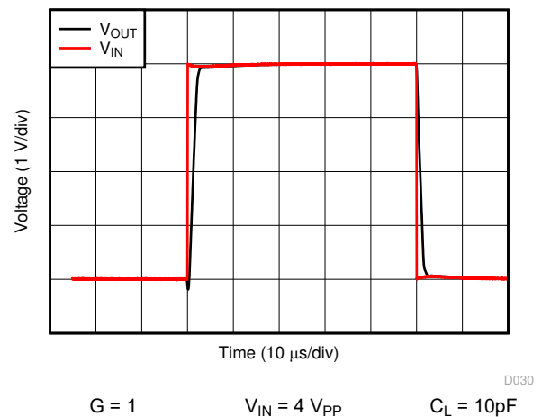
图 7-30. 大信号阶跃响应
