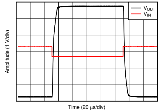
图 7-28. 过载恢复
