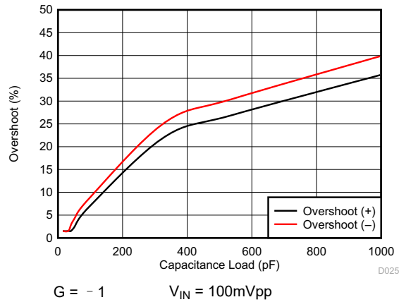
图 7-25. 小信号过冲与容性负载间的关系
