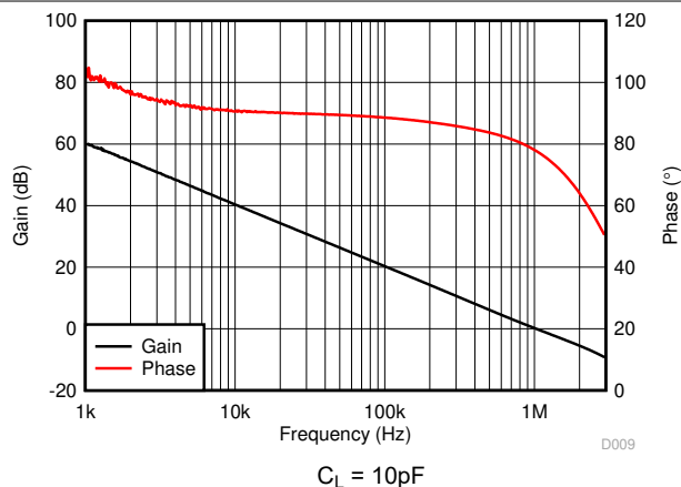
图 7-9. 开环增益和相位与频率间的关系
