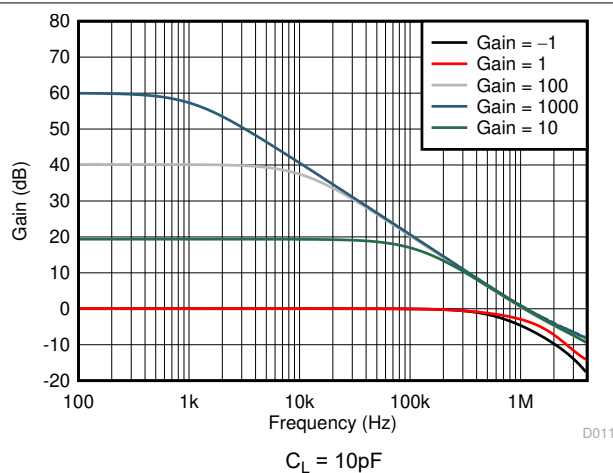
图 7-11. 闭环增益与频率间的关系
