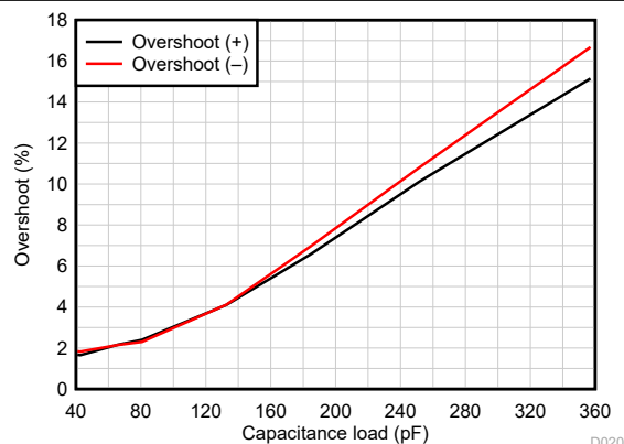
图 6-26. 小信号过冲与容性负载间的关系
