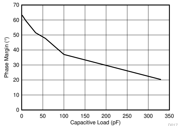
图 7-17. Phase Margin vs Capacitive Load
