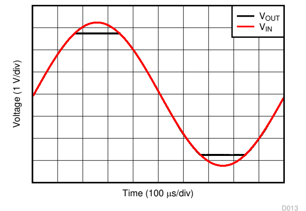
图 7-18. No Phase Reversal
