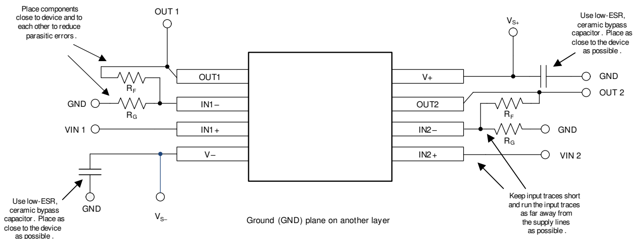
图 9-4. Layout Example
