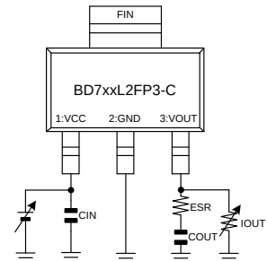
SOT223-4(F)
