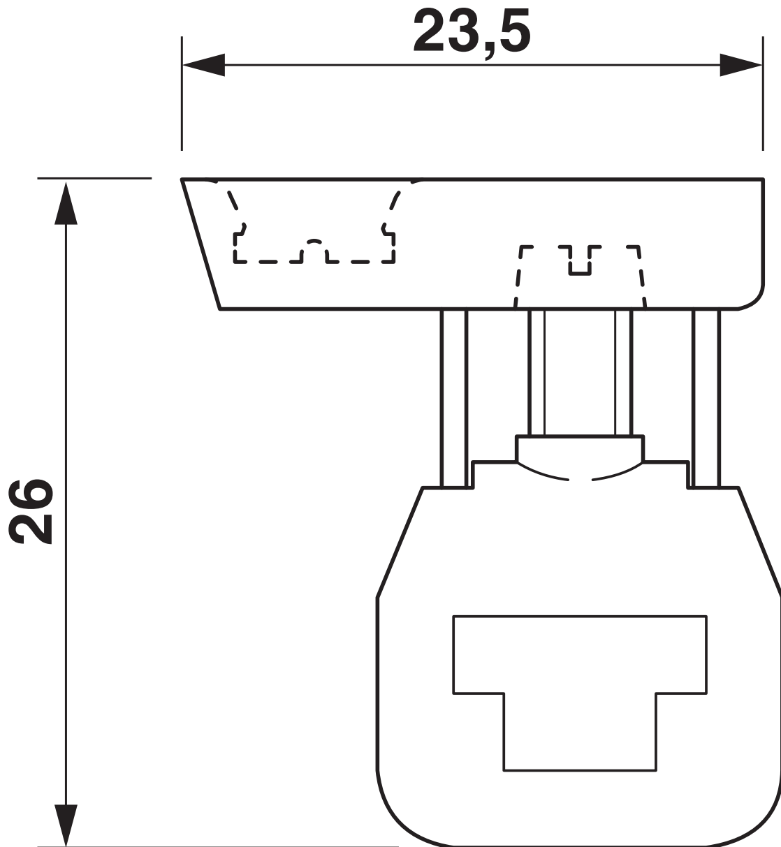
尺寸图
