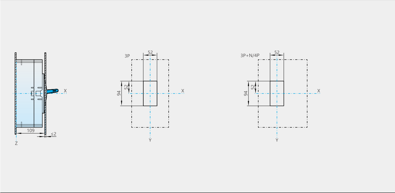
NXMLE-400S/H、630S/H 柜门开孔 (小) 尺寸 (mm)
