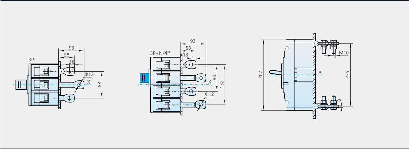
NXMLE-400S/H、630S/H 板后接线 外形尺寸 (mm)
