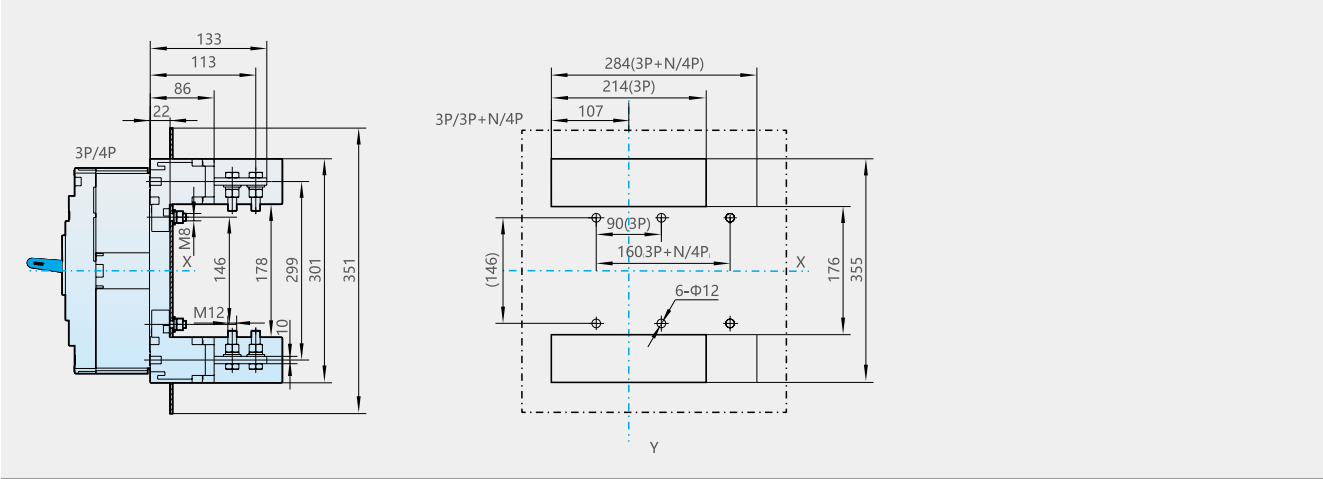
NXMLE-800S/H 插入式板后接线 外形及安装尺寸 (mm)
