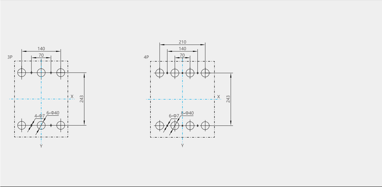
NXMLE-800S/H 板后接线 安装尺寸 (mm)
