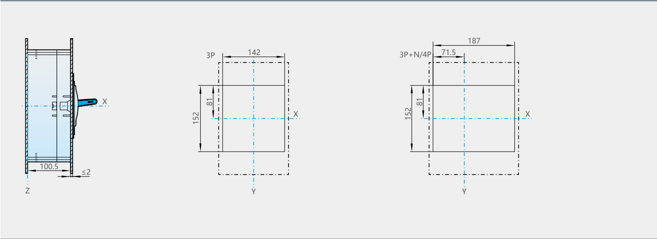
NXMLE-400S/H、630S/H 柜门开孔 (大) 尺寸 (mm)
