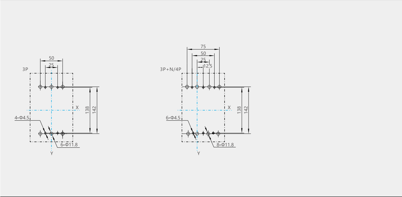
NXMLE-125S/H 板后接线 安装尺寸 (mm)
