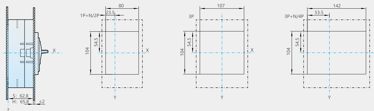
柜门开孔 (大) 尺寸 (mm)
