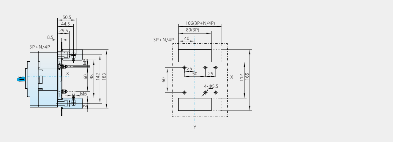
NXMLE-125S/H 插入式板后接线 外形及安装尺寸 (mm)
