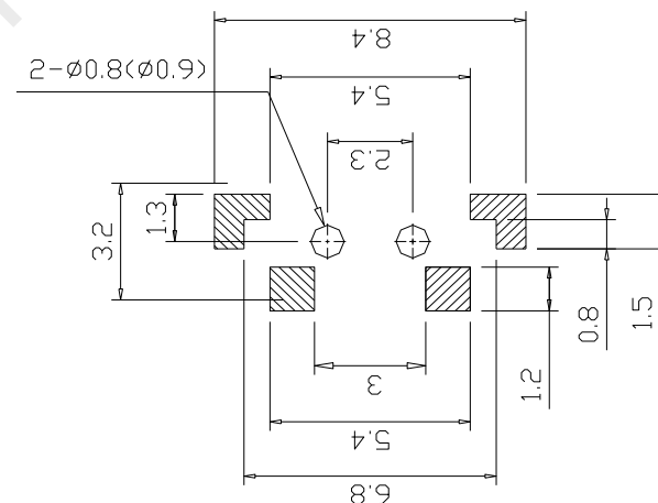
PCB. 焊接图
