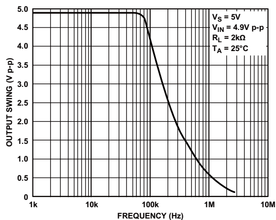
图24. 闭环输出电压摆幅与频率的关系
