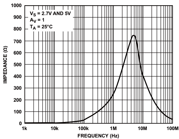
图34. 闭环输出阻抗与频率的关系
