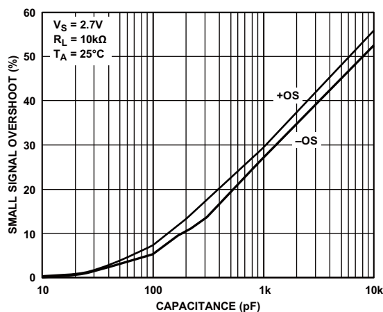
图14. 小信号过冲与负载电容的关系
