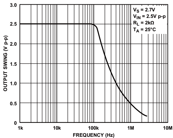
图12. 闭环输出电压摆幅与频率的关系
