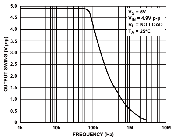
图23. 闭环输出电压摆幅与频率的关系
