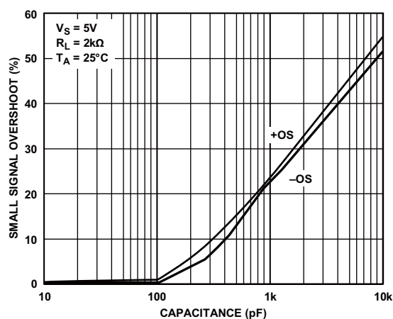
图26. 小信号过冲与负载电容的关系
