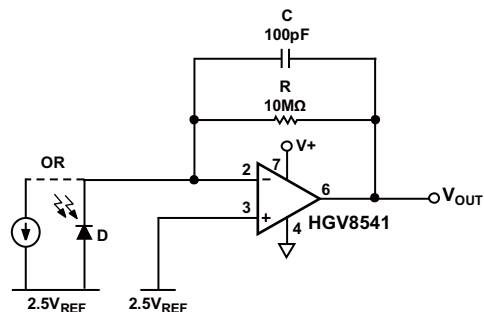
图40. 高输入阻抗应用——光电二极管放大器
