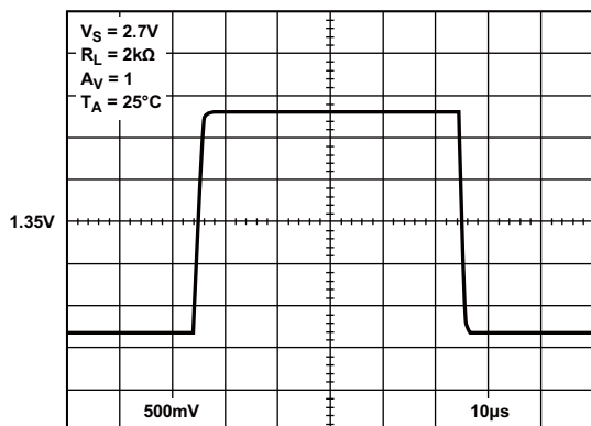
图17. 大信号瞬态响应
