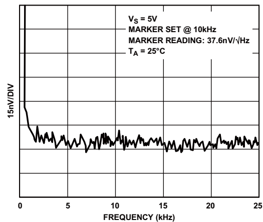
图35. 电压噪声
