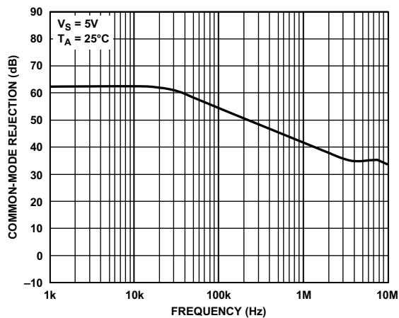
图20. 共模抑制与频率的关系
