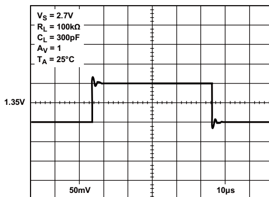
图16. 小信号瞬态响应
