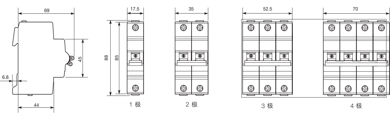
M200M 外形尺寸 (与S200系列一致)
