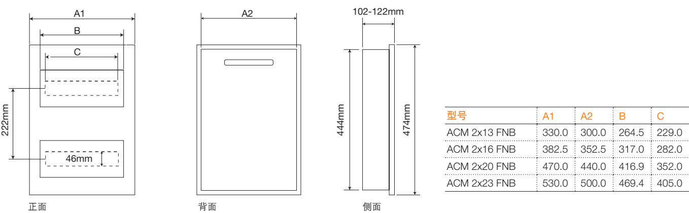
暗箱 ACM ... FNB 系列（双排标准暗箱）
