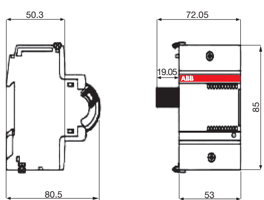
自动重合装置 - F2C - ARH
