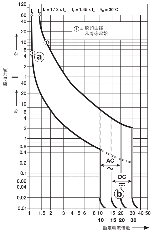
脱扣特性 D IEC-60898
