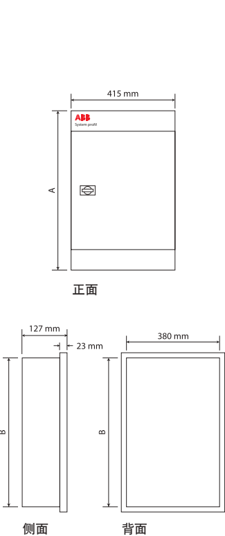
SDB-FB ( 嵌墙式安装 )
