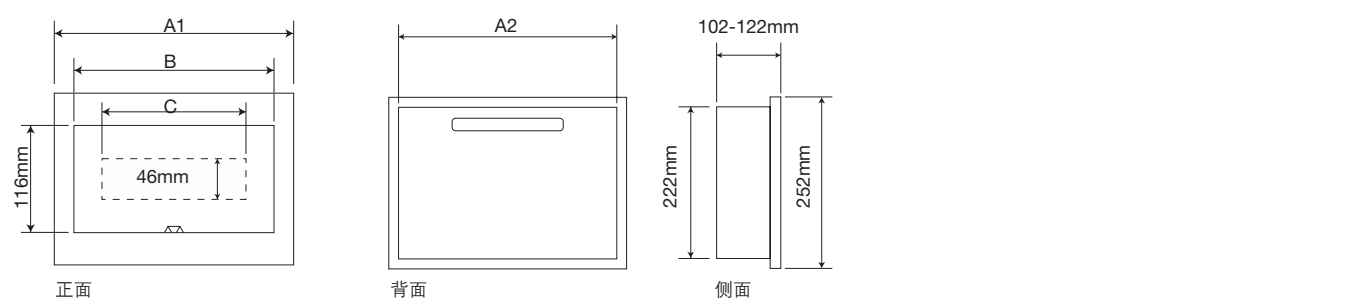
暗箱 ACM ... FNB 和 ACP ... FNB 系列
