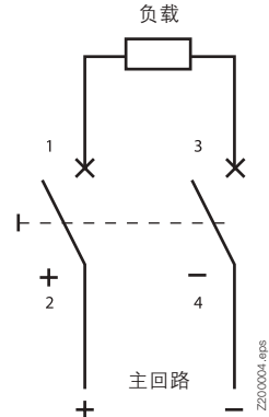
接线图
