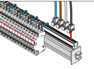
母排采用 100A 供电套件供电（不带电缆）。端子接线能力 35mm²。
