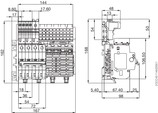
基座 (ZLS908) (8 模数)
