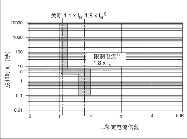
时间/电流特性曲线 ( T_U = 25^\circ C )
