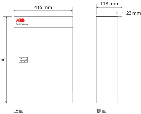
SDB - SEB（挂墙式）
