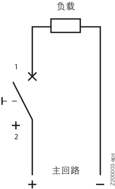
接线图 单极 (max. 125 V=) S401M-UCC
