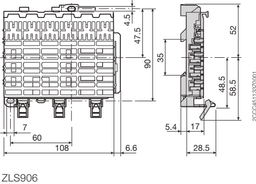
基座 (ZLS906) (6 模数)
