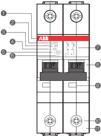
正面 1 品牌标识 2 断路器系列和极数 3 脱扣特性及额定电流 4 额定电压 5 分断能力 6 限流等级 7 接线图 8 操作手柄 9 CPI 触头位置指示器 - 红色 ON 闭合状态 - 绿色 OFF 断开状态 10 紧固螺钉 11 外壳
