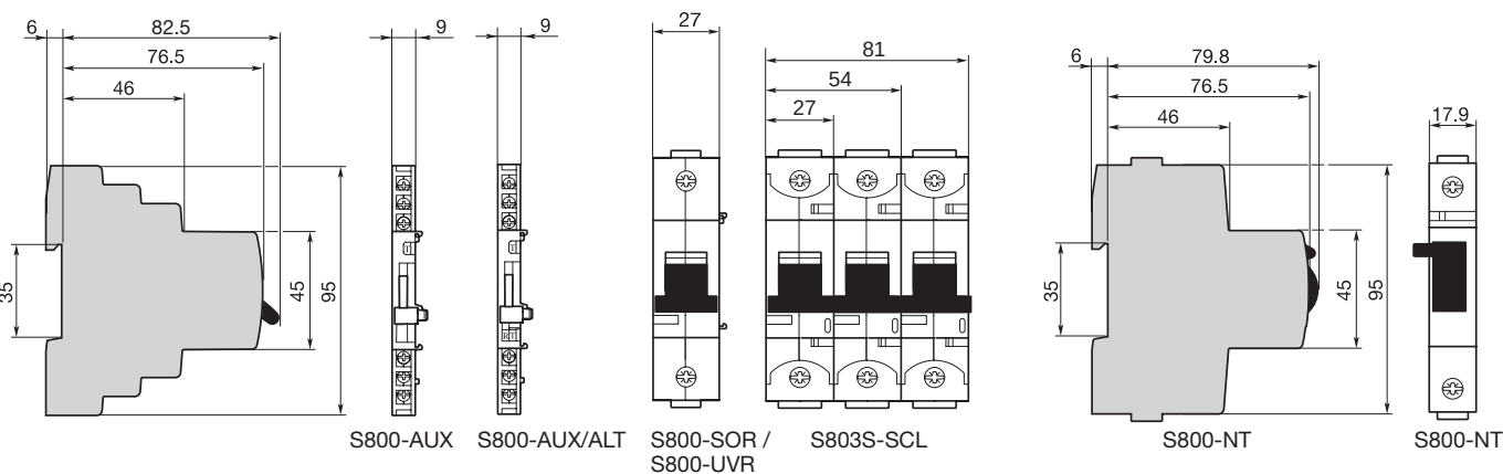
S800 辅件及附件
