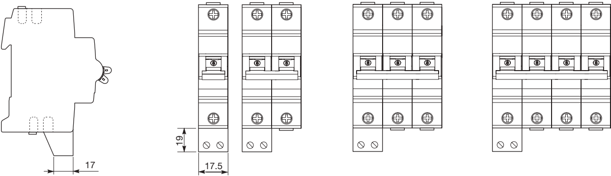
辅助触头（安装在 S200 底部 - S2C - H10 / H01）
