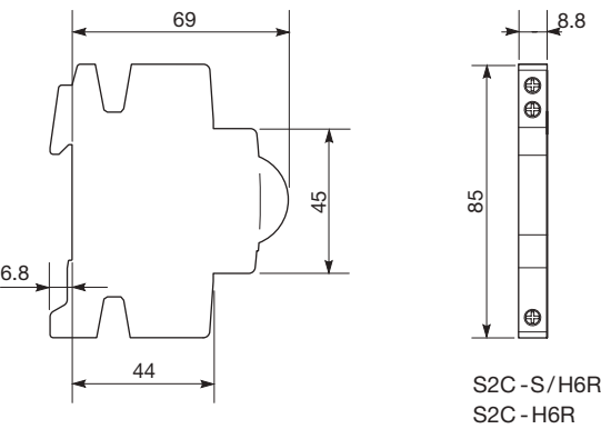
辅助触头 / 信号辅助触头
