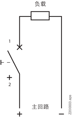
接线图 单极 (max. 125 V=) S401M-UCZ
