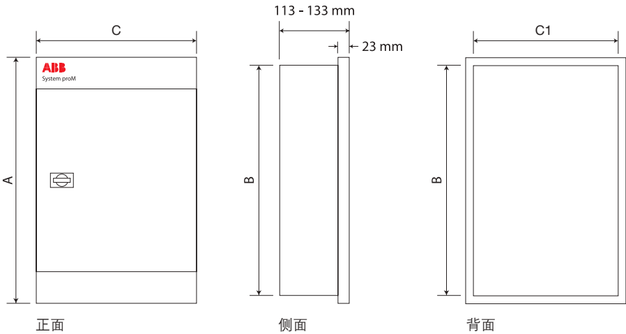
SDB - SEBF（嵌墙式）
