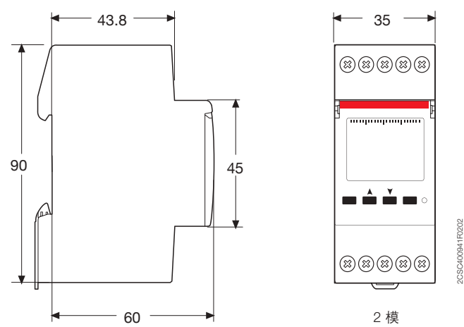
D Line 数字式定时器
