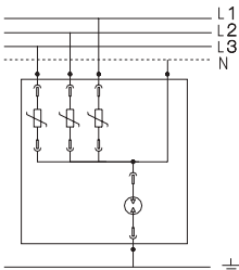
OVR BT2 3N...P
