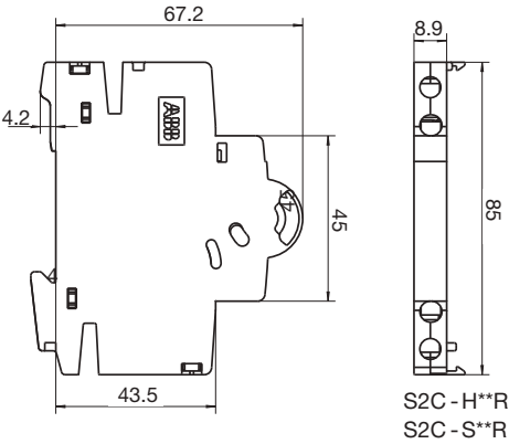
辅助触点 / 信号触点
