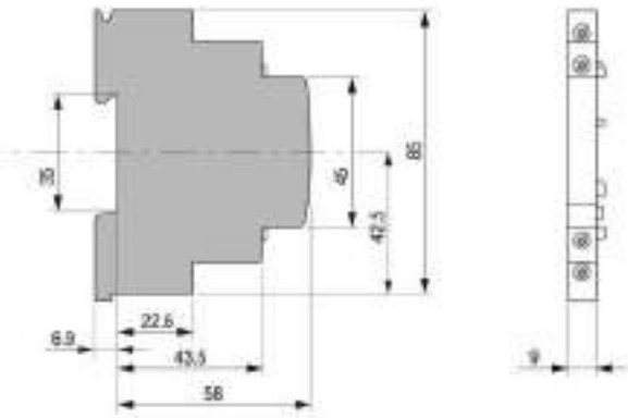
E293/X中央控制模块 （相同控制电压）
