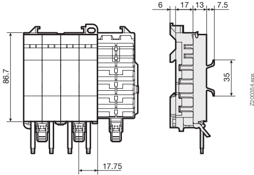
通用适配器 (32 A, 63 A)
