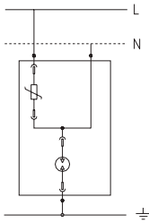
OVR BT2 1N...P
