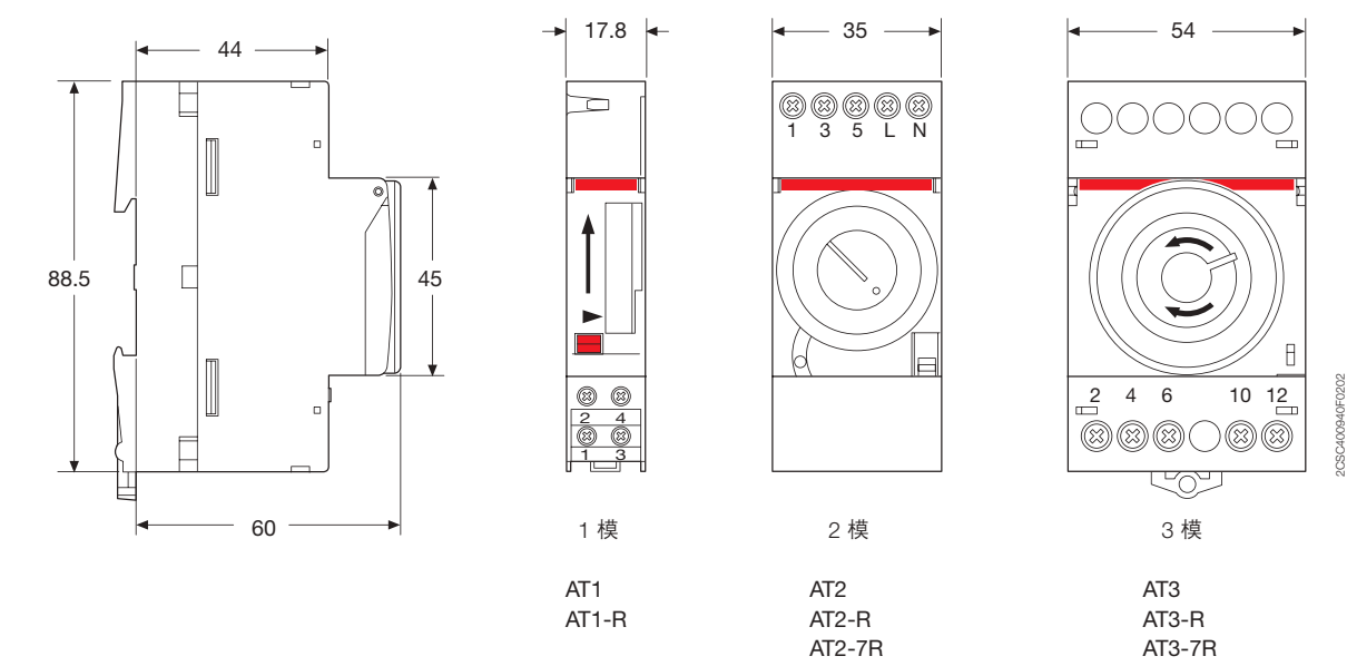
AT 机械式定时器
