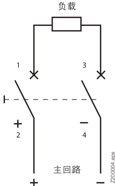
接线图 2极 (max. 250 V=) S402M-UCZ
