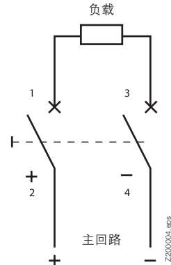
接线图 2极 (max. 250 V=) S402M-UCC
