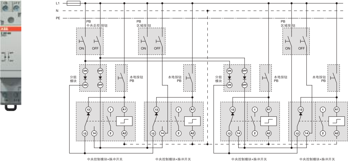
E290-16-10 + E293/X + E295-GM — 脉冲开关与中央控制模块和分组模块配合使用
