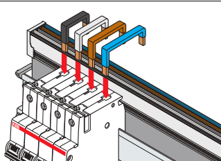
System Pro M 系列模数化装置的连接 (L1-L2-L3-N)。
