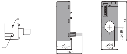
互感器 (CMS-100PS)
