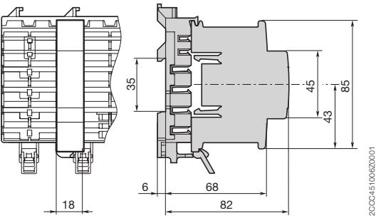
填充片 (ZLS 725)
