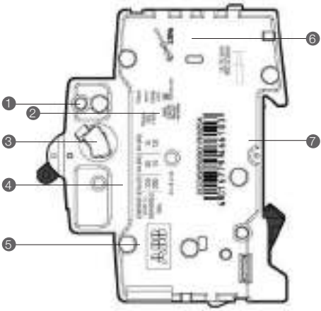
右侧面 1 附件安装孔 2 认证标志 3 多极连接孔 4 试验参数 5 品牌标识 6 最大拧紧力矩 7 产品条码
