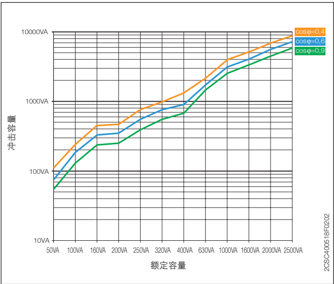
冲击容量
