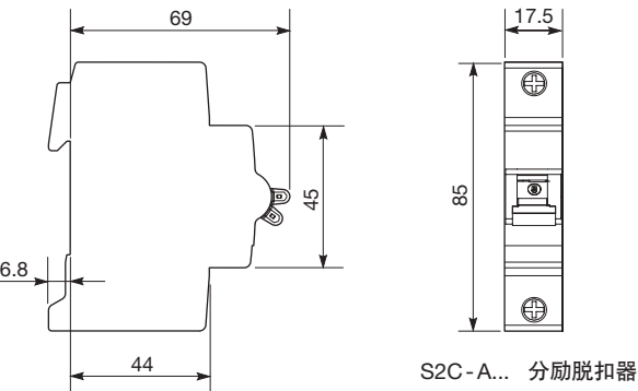
分励脱扣器 / 欠电压脱扣器 / 过电压脱扣器
