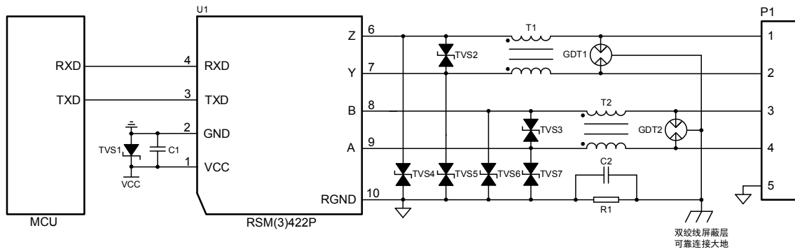
图 2 推荐应用电路 2
