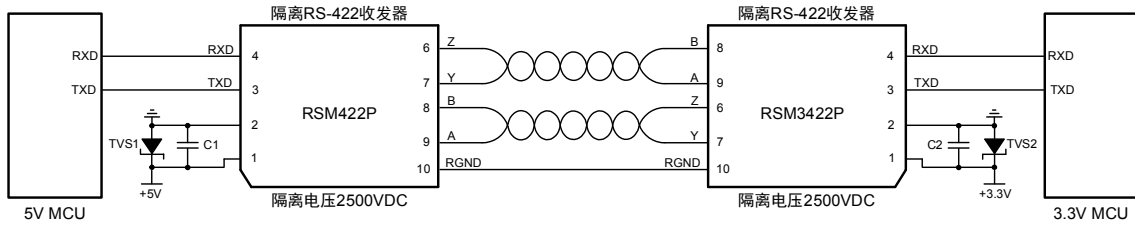
图 1 点对点连接电路图
