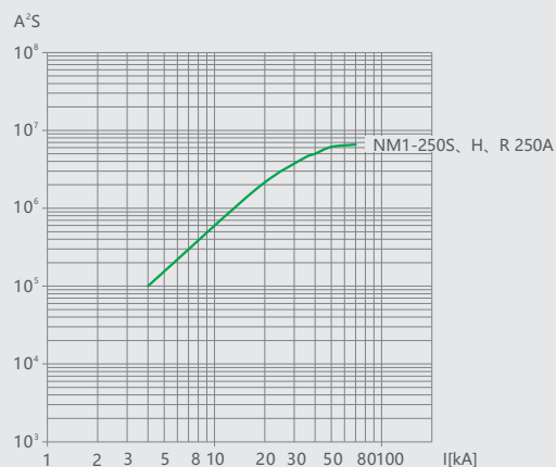
图40 NM1-250 允通曲线
