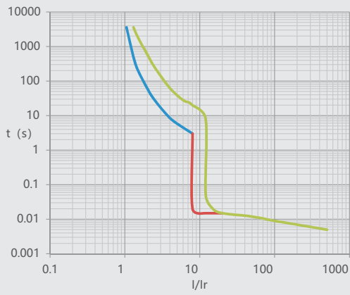
图15 NM1-125 32A-63A电动机保护
