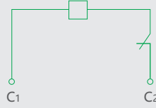
分励脱扣器接线图
