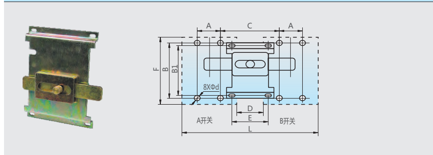
安装尺寸图(见表15)
