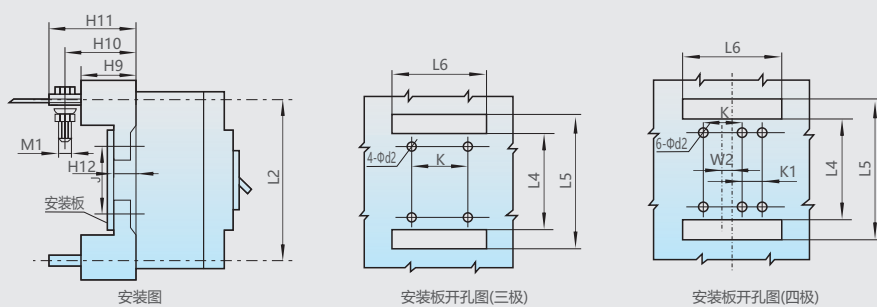
安装图
