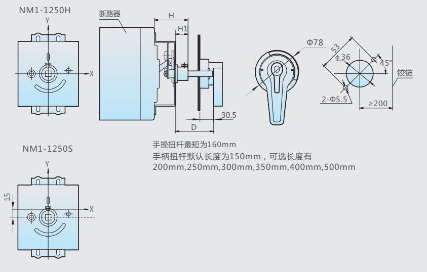
NM1-1250手柄安装开孔示意图
