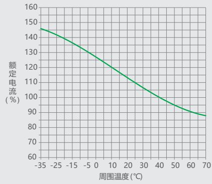
图32 NM1-800 温度补偿曲线
