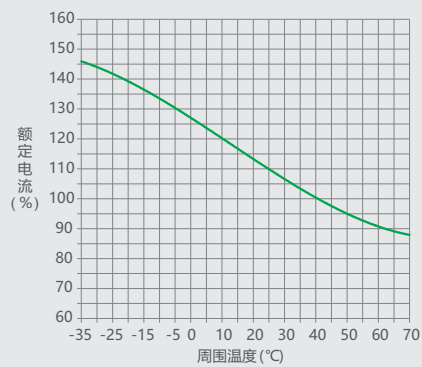
图34 NM1-800 温度补偿曲线
