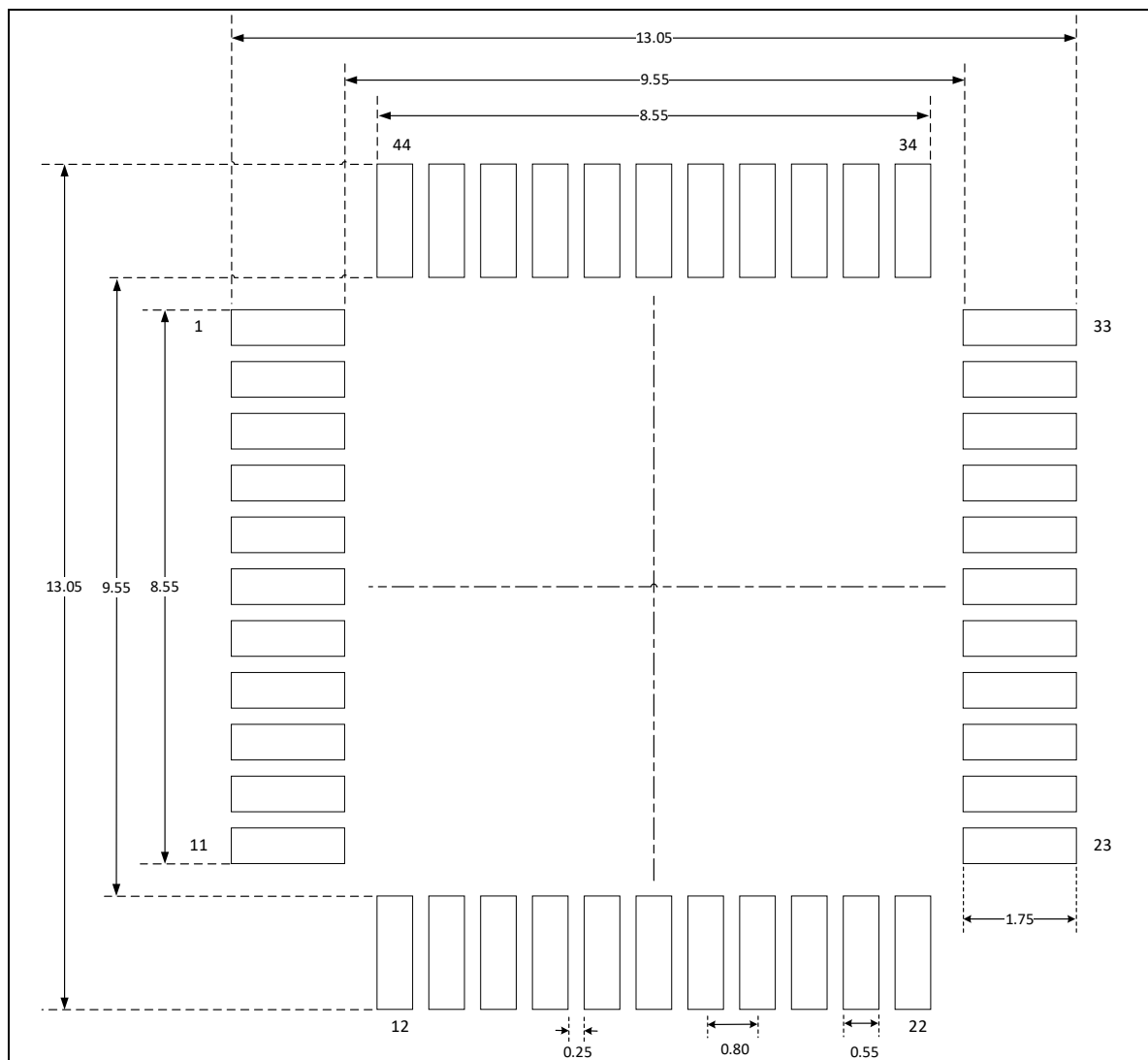
LQFP44 封装 (10mm x 10mm)
