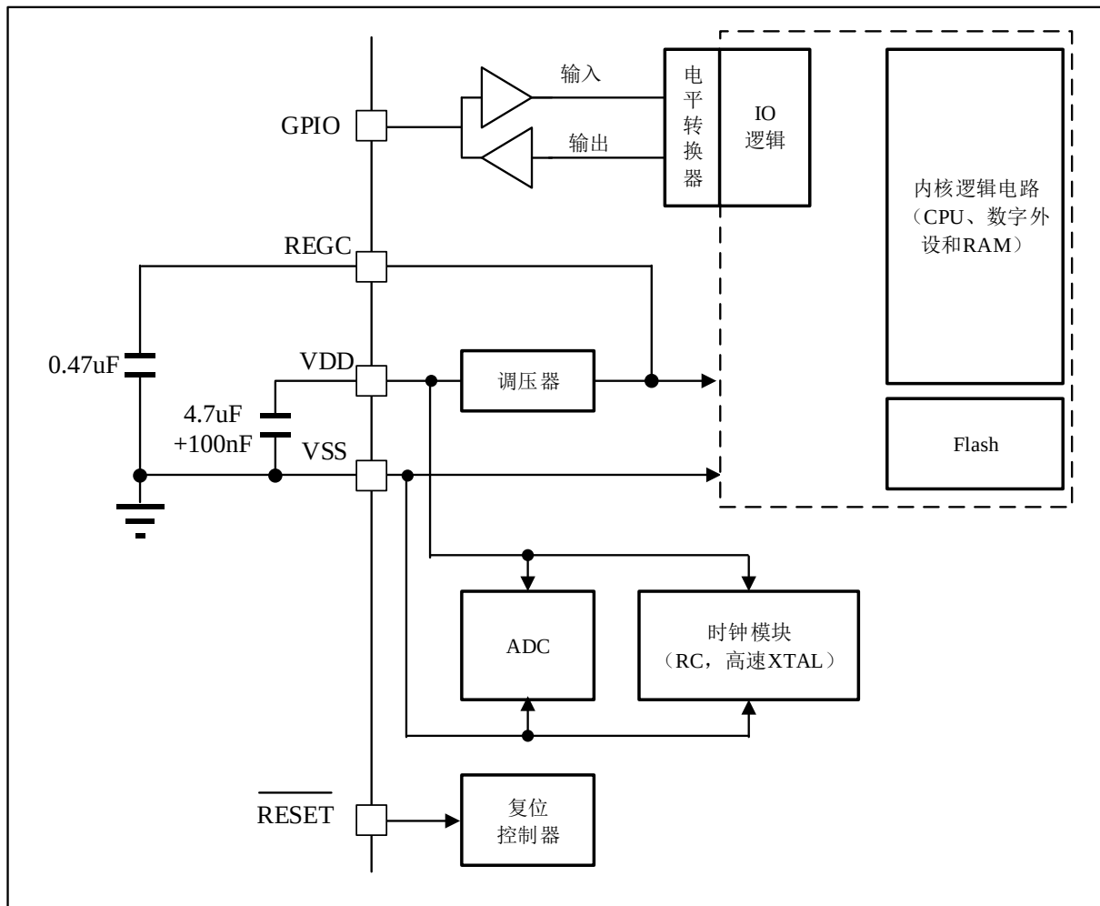
图 3-2 电源方案
