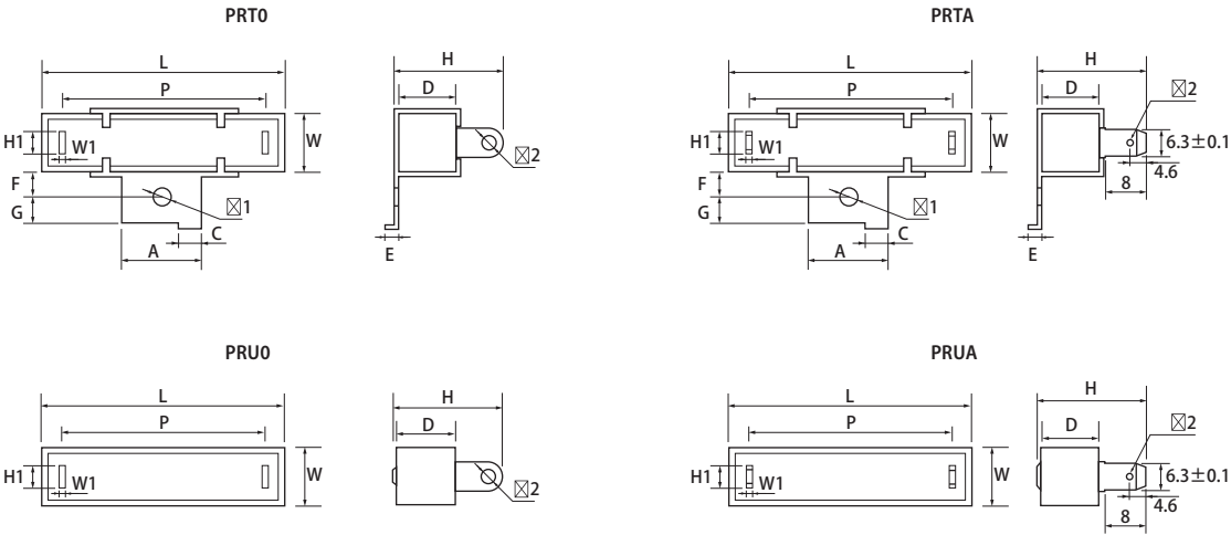
立式端片型 PRT (带金属安装支架)/PRU
