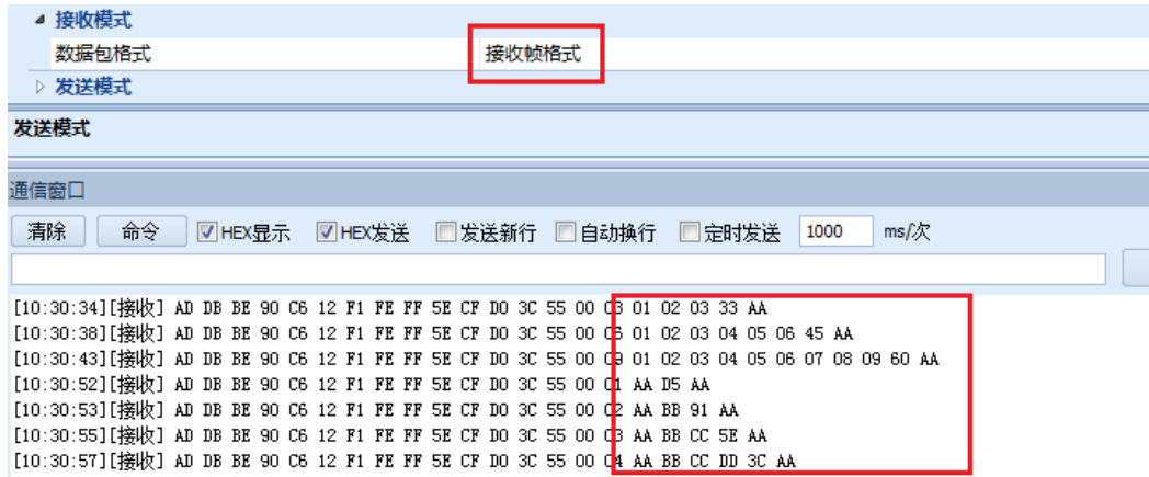
图 8.5 接收帧
