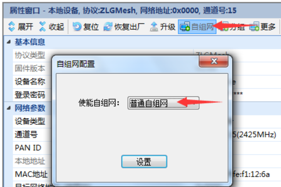
图 6.5 配置自组网
