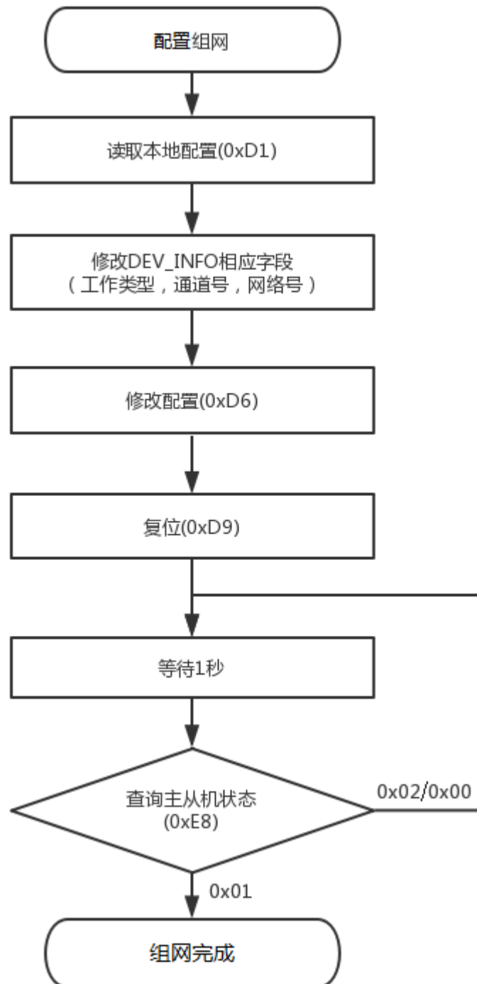
图 15.1 配置组网
