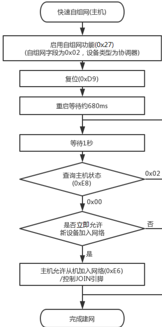
图 15.4 快速自组网-主机
