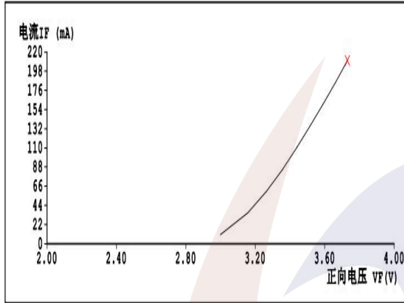
电压与电流
