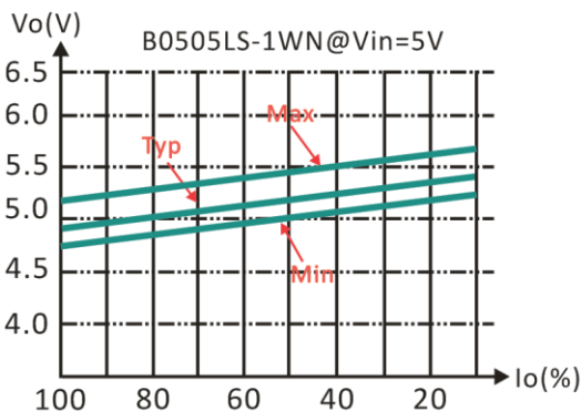
输出电压VS负载关系曲线
