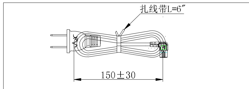
扎线示意图:
