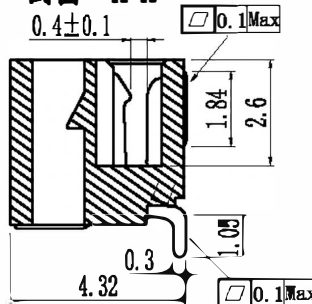
剖面 A-A
