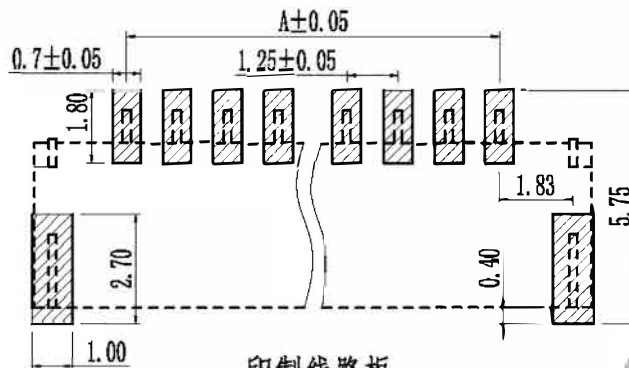
印制线路板
