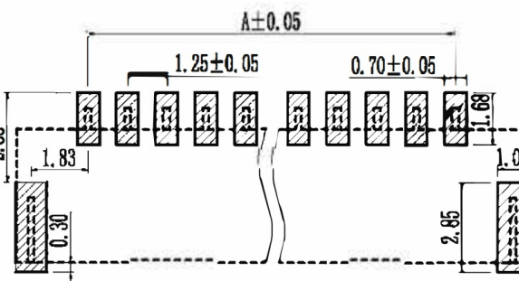
印制线路板
