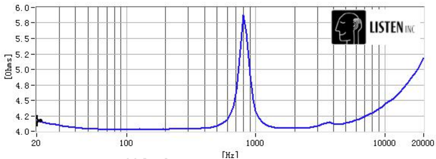
阻抗曲线
