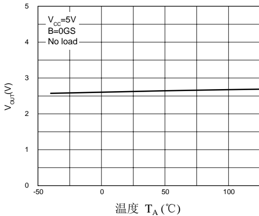
静态输出电压随温度的变化
