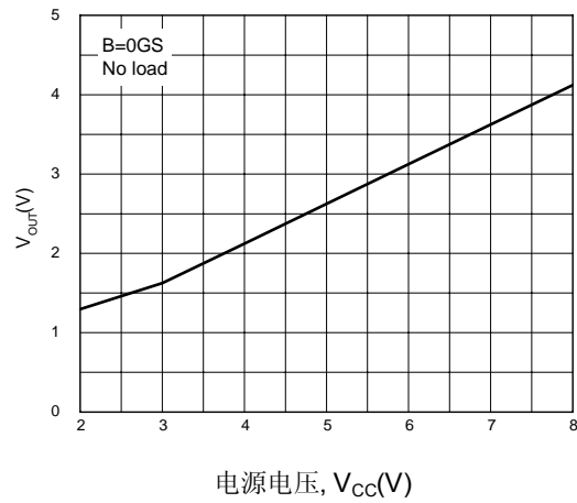
静态输出电压随电源电压的变化
