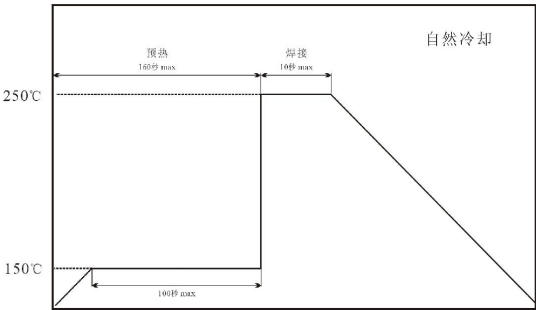
锡铅产品回流焊曲线 (Sn/Pb product)
